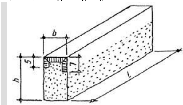
Krawężnik drogowy rodzaju A
