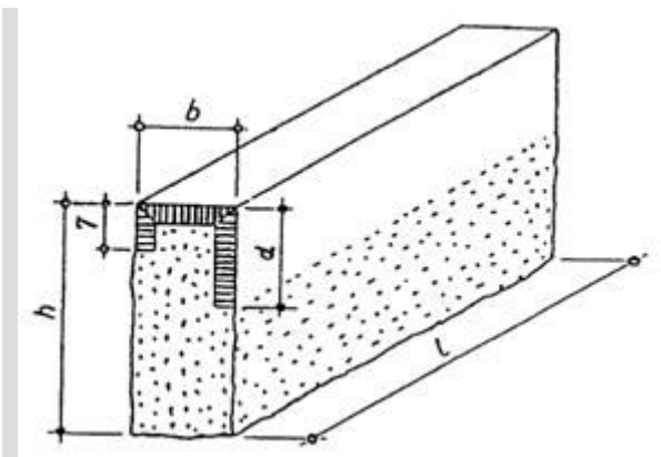
Krawężnik uliczny rodzaju B
