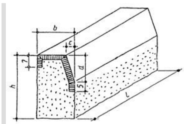
Krawężnik uliczny rodzaju A
